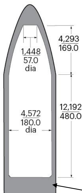
Coiffe de l'Atlas V-541
