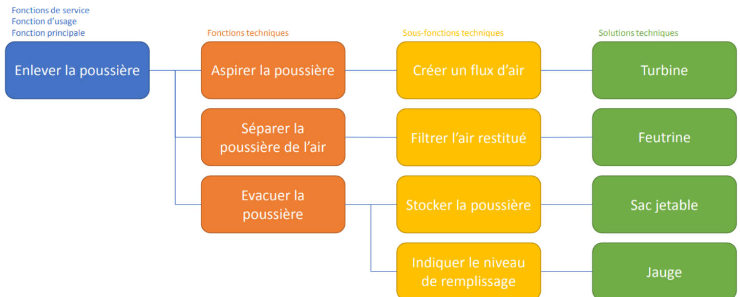
Diagramme FAST
